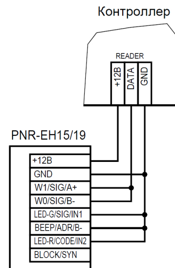
Рисунок 8. Подключение считывателя по интерфейсу Touch Memory
