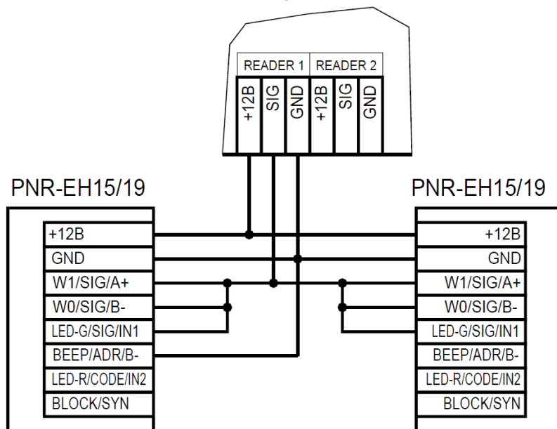
Рисунок 12. Подключение двух считывателей по интерфейсу Parsec одним кабелем
