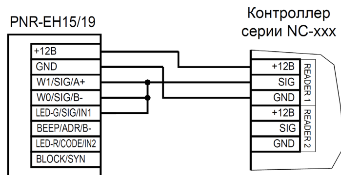
Рисунок 10. Подключение считывателя по интерфейсу Parsec, адрес 1 (внутренний)
