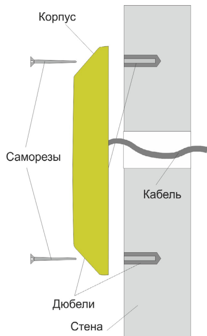
Рисунок 2. Крепление PR-M03
