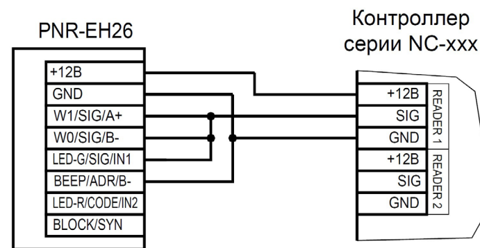
Рисунок 10. Подключение считывателя по интерфейсу Parsec, адрес 0 (наружный)
