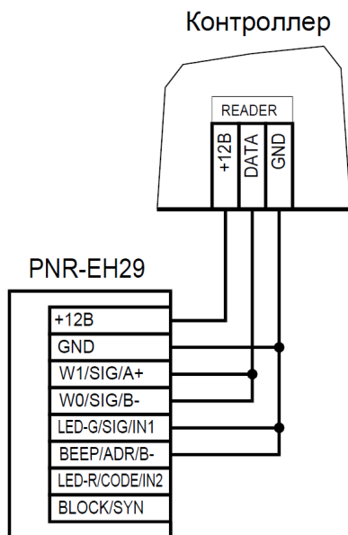
Рисунок 9. Подключение считывателя по интерфейсу Touch Memory
