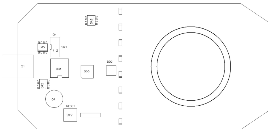
Рисунок 3. Плата считывателя PR-X18
