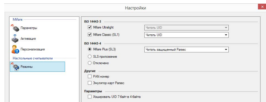
Рисунок 2. Настройки считывателя PR-P18 в ParsecNET 3
