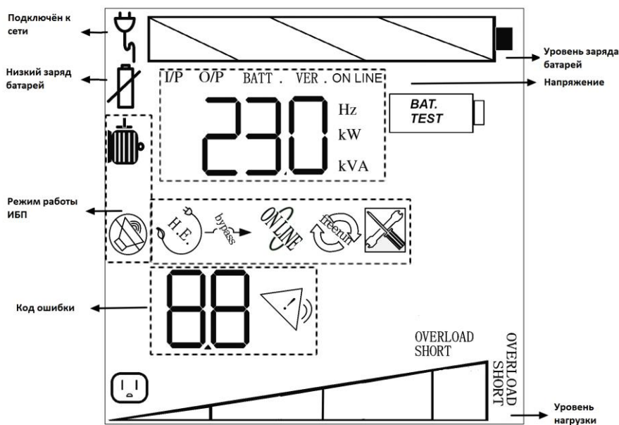
Рис. 7. ЖК-дисплей
