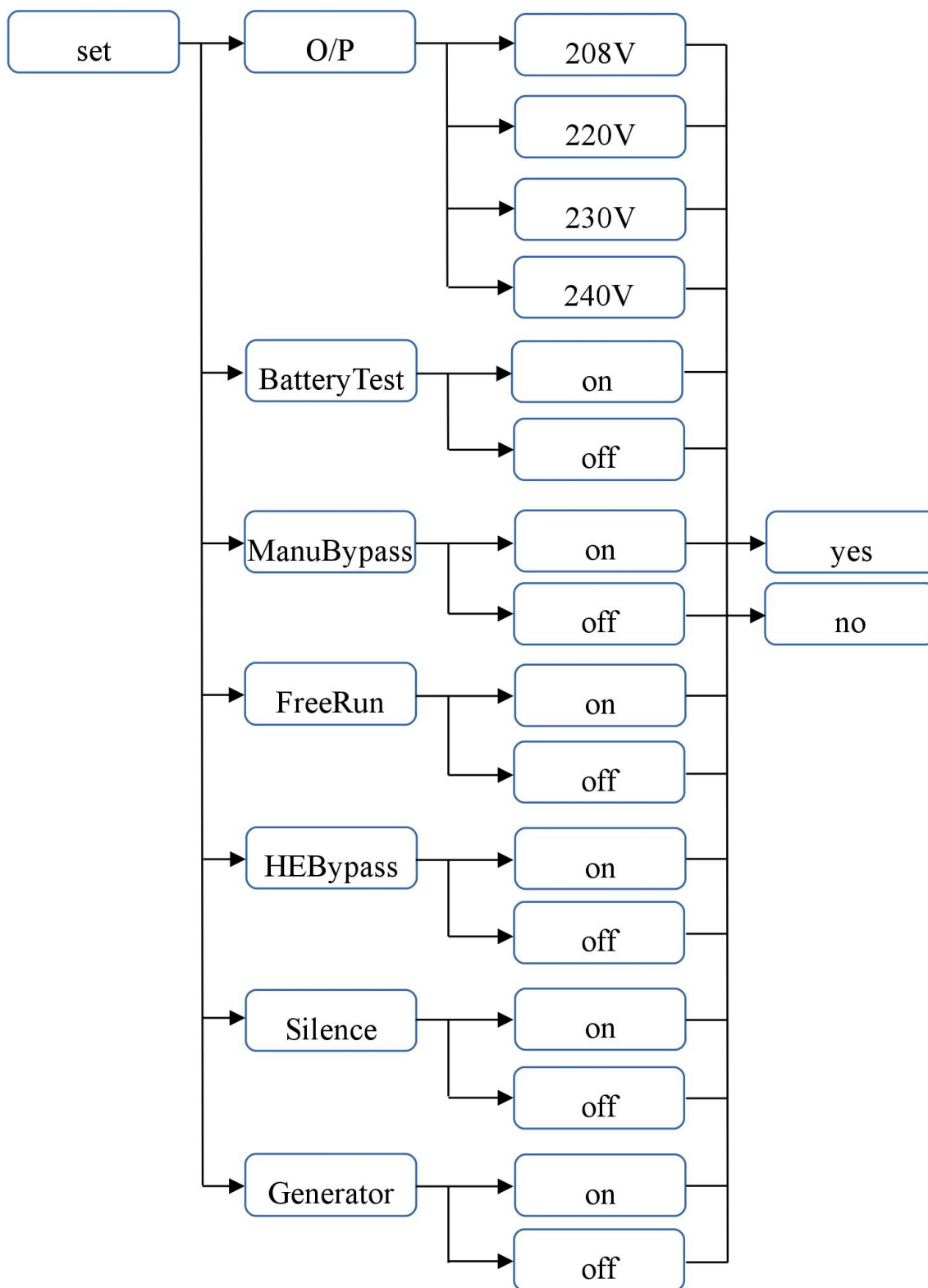
Рис. 9. Настройки ИБП
