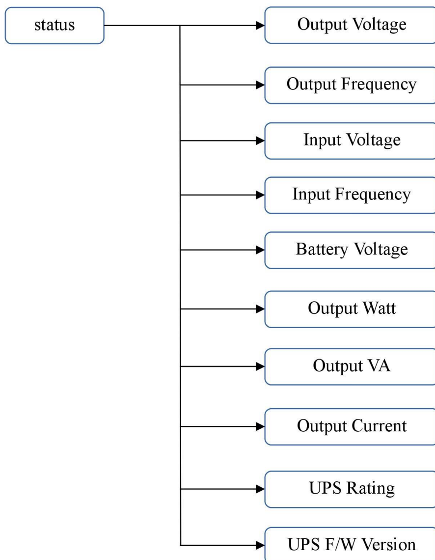
Рис. 8. Состояние ИБП
