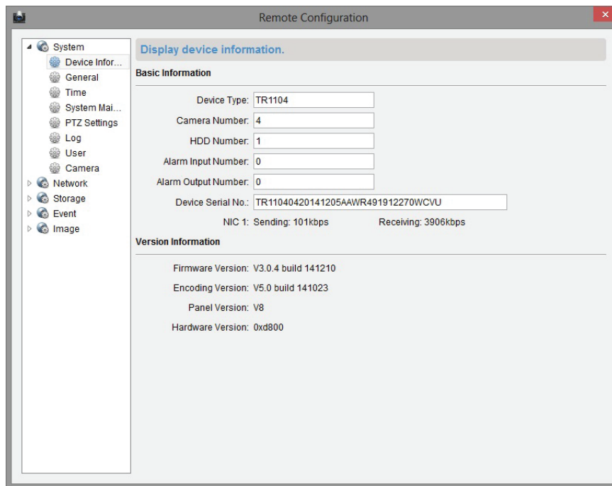
Рис. 87 Основная информация о устройстве
