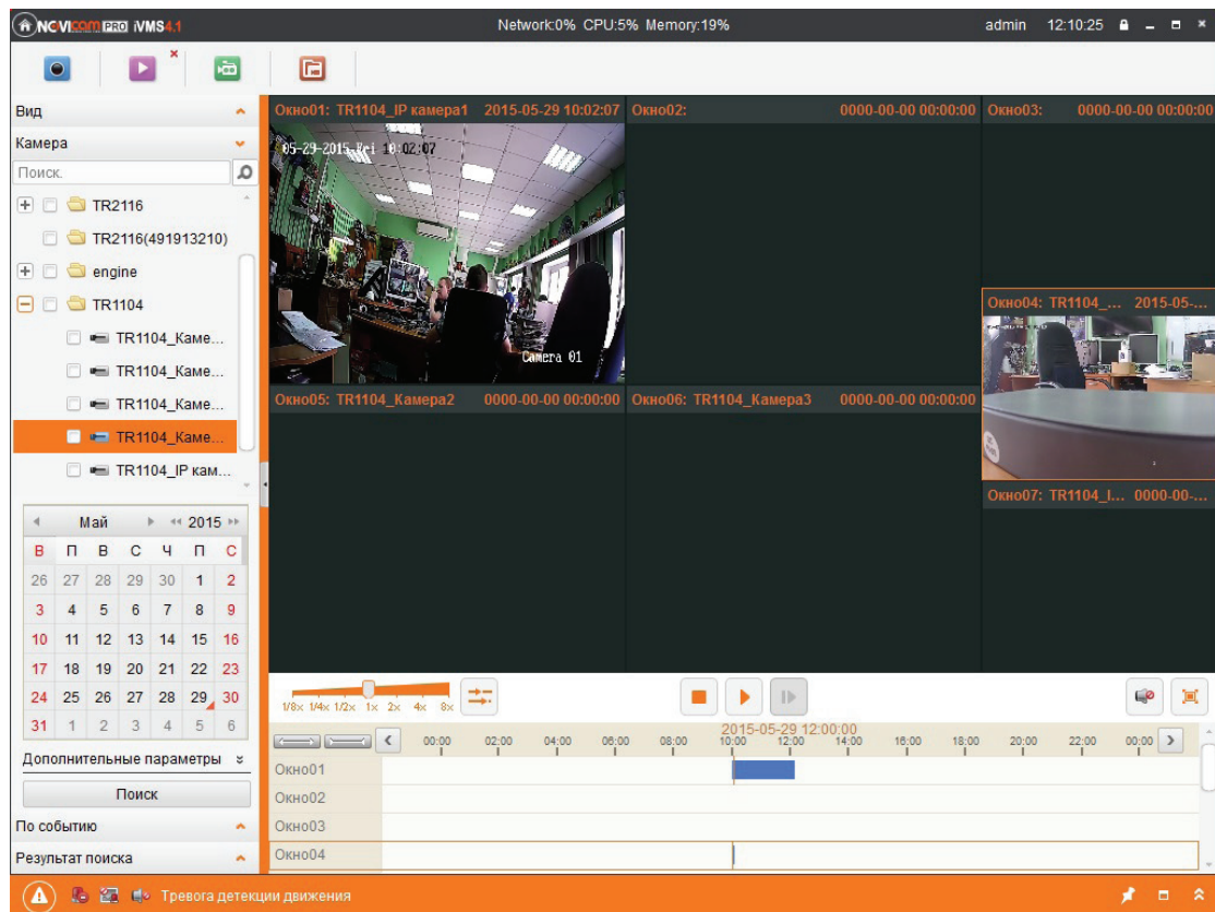
Рис. 84 Интерфейс воспроизведения
