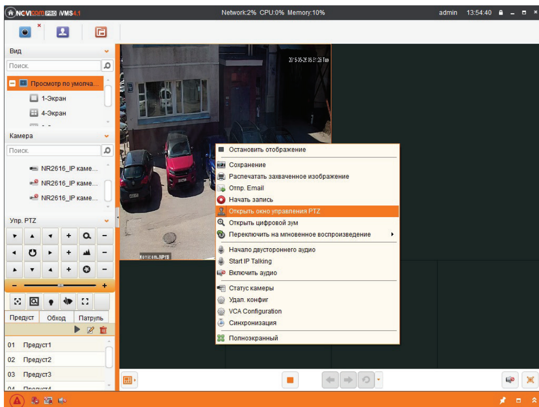
Рис. 31 Управление PTZ
