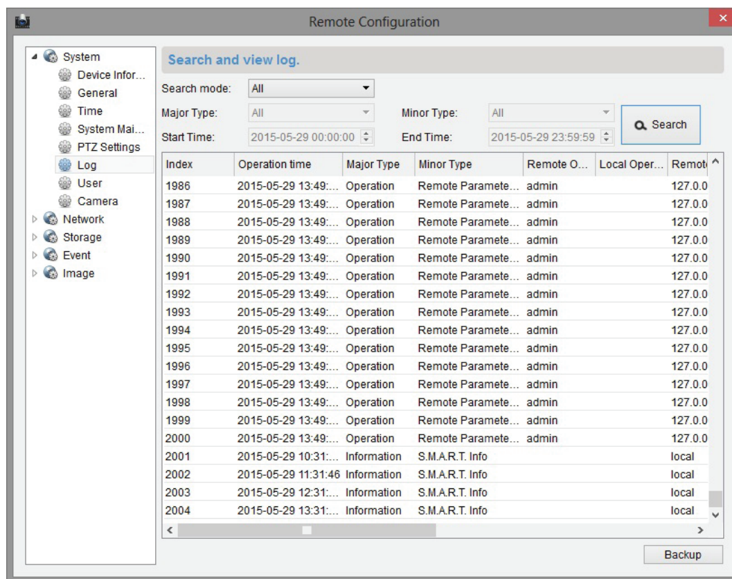
Рис. 99 Управление журналом
