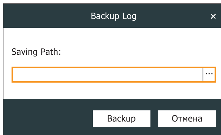
Рис. 124 Копирование журнала
