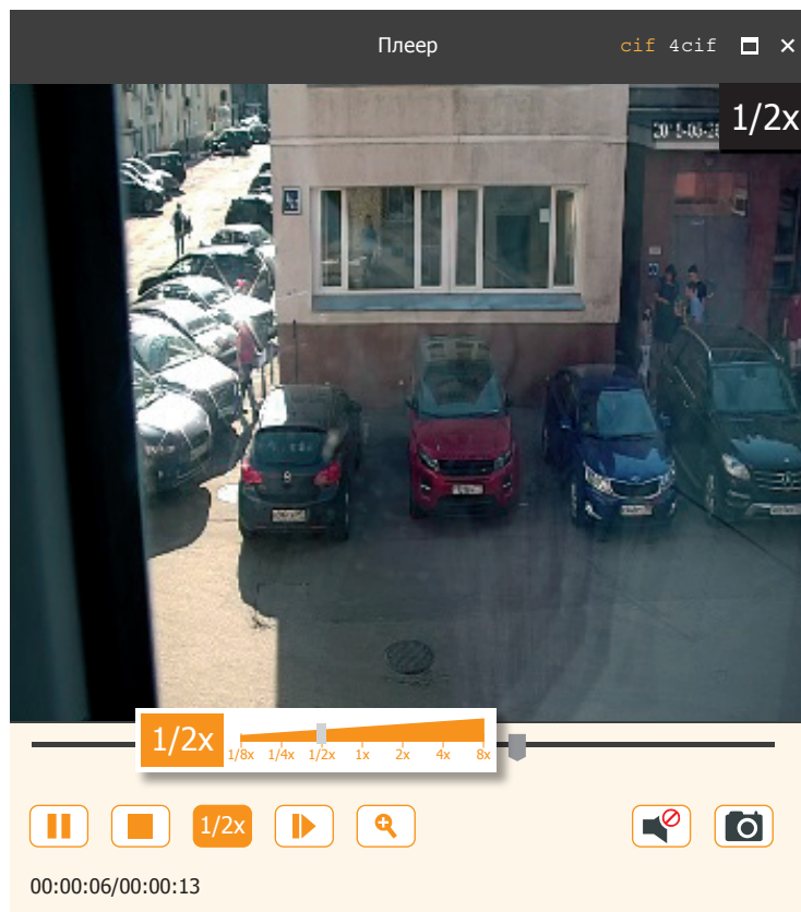
Рис. 45 Плеер
