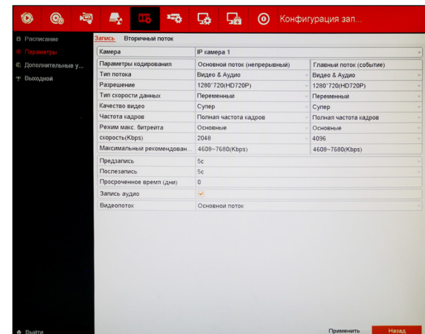
Рисунок 5.35 Настройка параметров записи основного потока.
