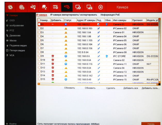
Рисунок 4.10 Добавление IP камер.
