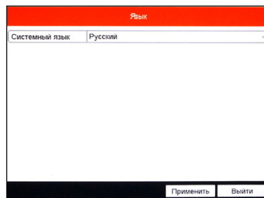
Рисунок 4.1 Выбор языка.
