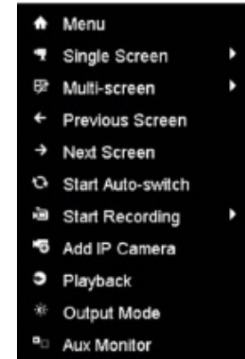
Рисунок 4.9 Всплывающее меню.
