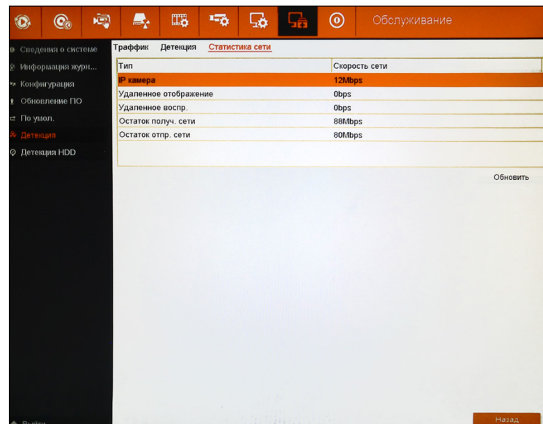
Рисунок 5.110 Статистика сети.
