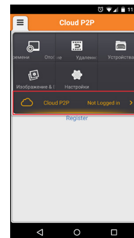
Рисунок 6.4 Cloud P2P.
