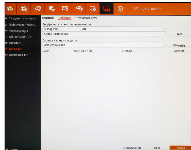
Рисунок 5.108 Детекция сети.
