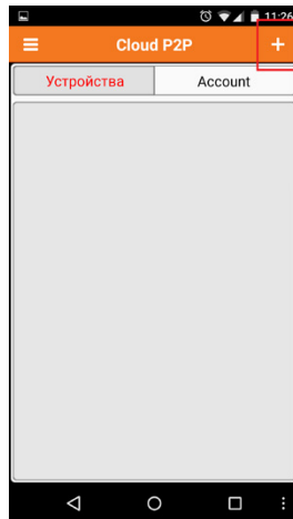
Рисунок 6.6 Устройства.
