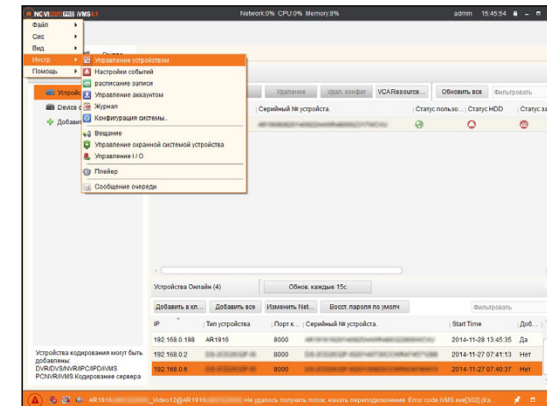
Рисунок 6.8 Управление устройством.
