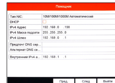
Рисунок 4.5 Настройка сети.
