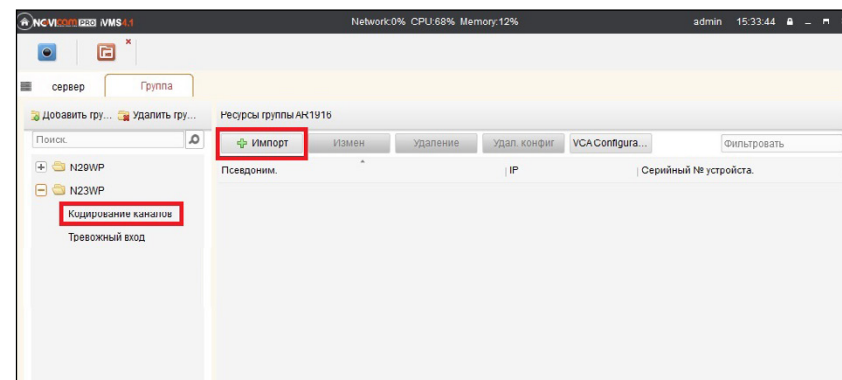
Рисунок 6.15 Импорт камеры.
