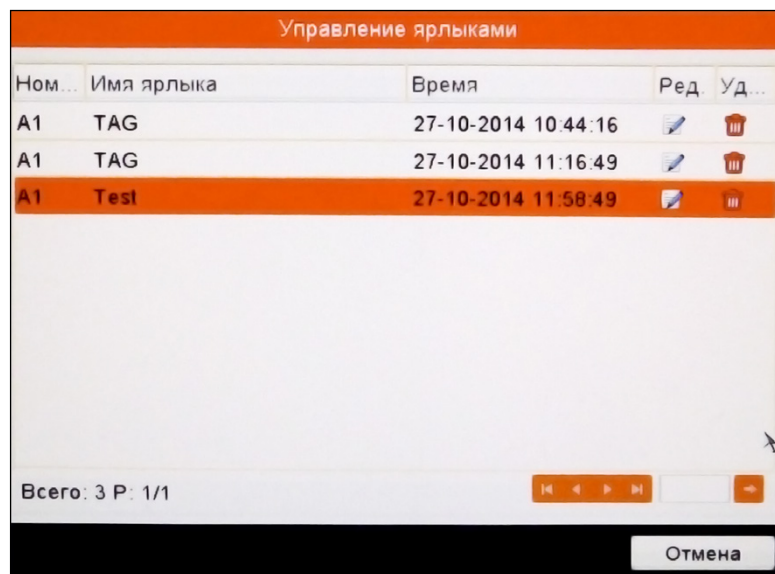
Рисунок 5.8 Управление ярлыками.
