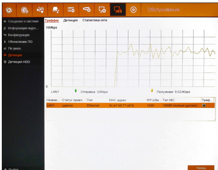
Рисунок 5.107 Трафик сети.
