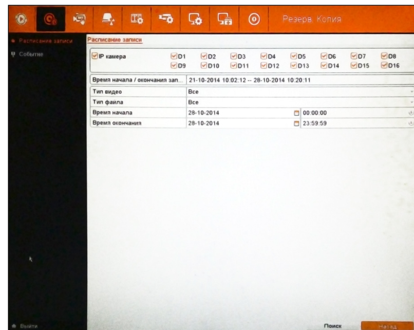
Рисунок 5.1 Расписание записи.
