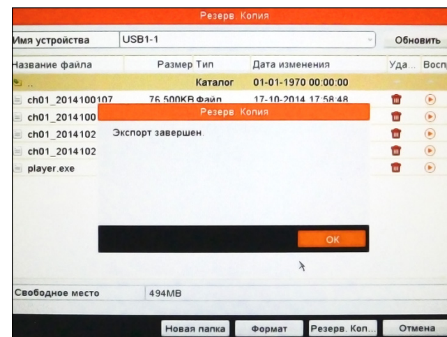
Рисунок 5.7 Экспорт завершён.
