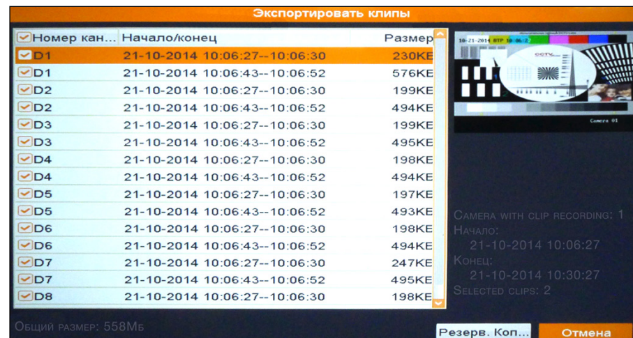
Рисунок 5.5 Копирование клипов.
