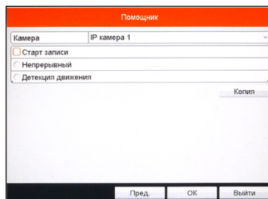
Рисунок 4.8 Настройка записи.
