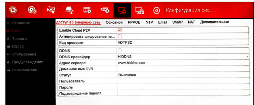
Рисунок 6.1 Активация облака.
