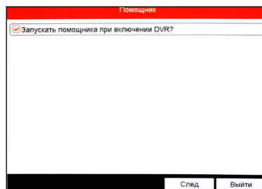
Рисунок 4.2 Активация помощника.
