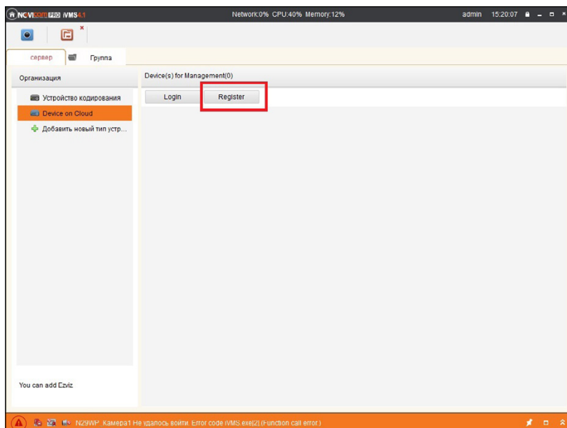
Рисунок 6.10 Регистрация.
