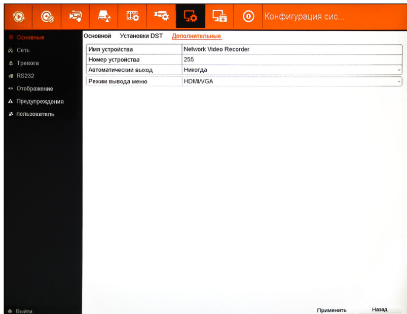
Рисунок 5.68 Дополнительные настройки.
