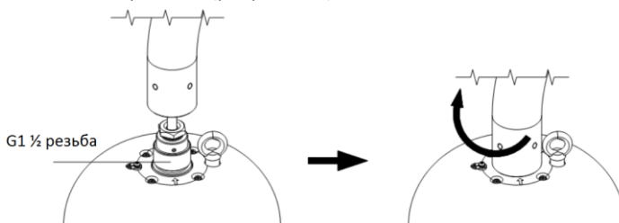
Рисунок 2-8 Установка кронштейна
