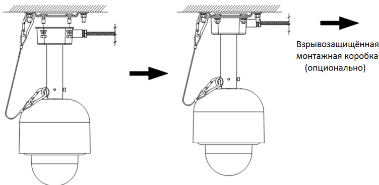
Рисунок 2-11 Закрепление кронштейна
