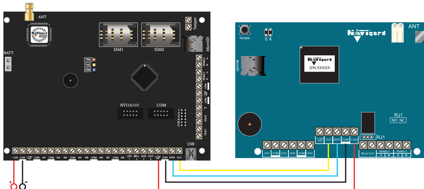
Рисунок 23. Подключение клавиатуры 8500
