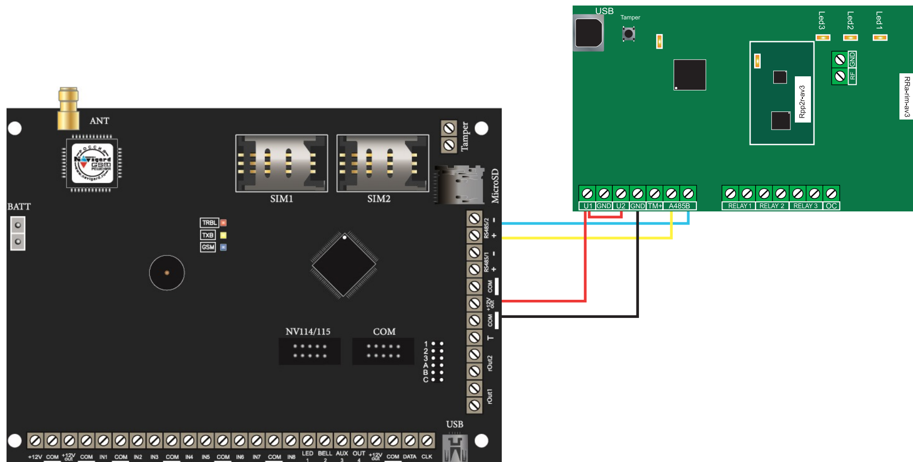
Рисунок 22. Подключение радиорасширителя Астра PI-M PP
