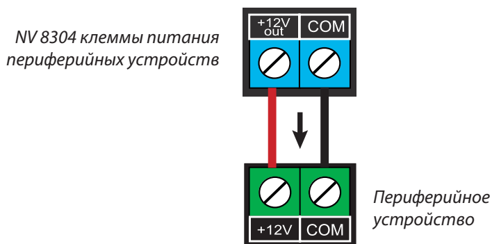
Подключение питания
