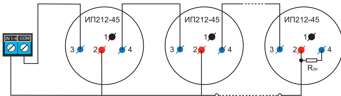
Схема подключения ИП212-45 к пожарному входу NV 8304 только с оконечным резистором
