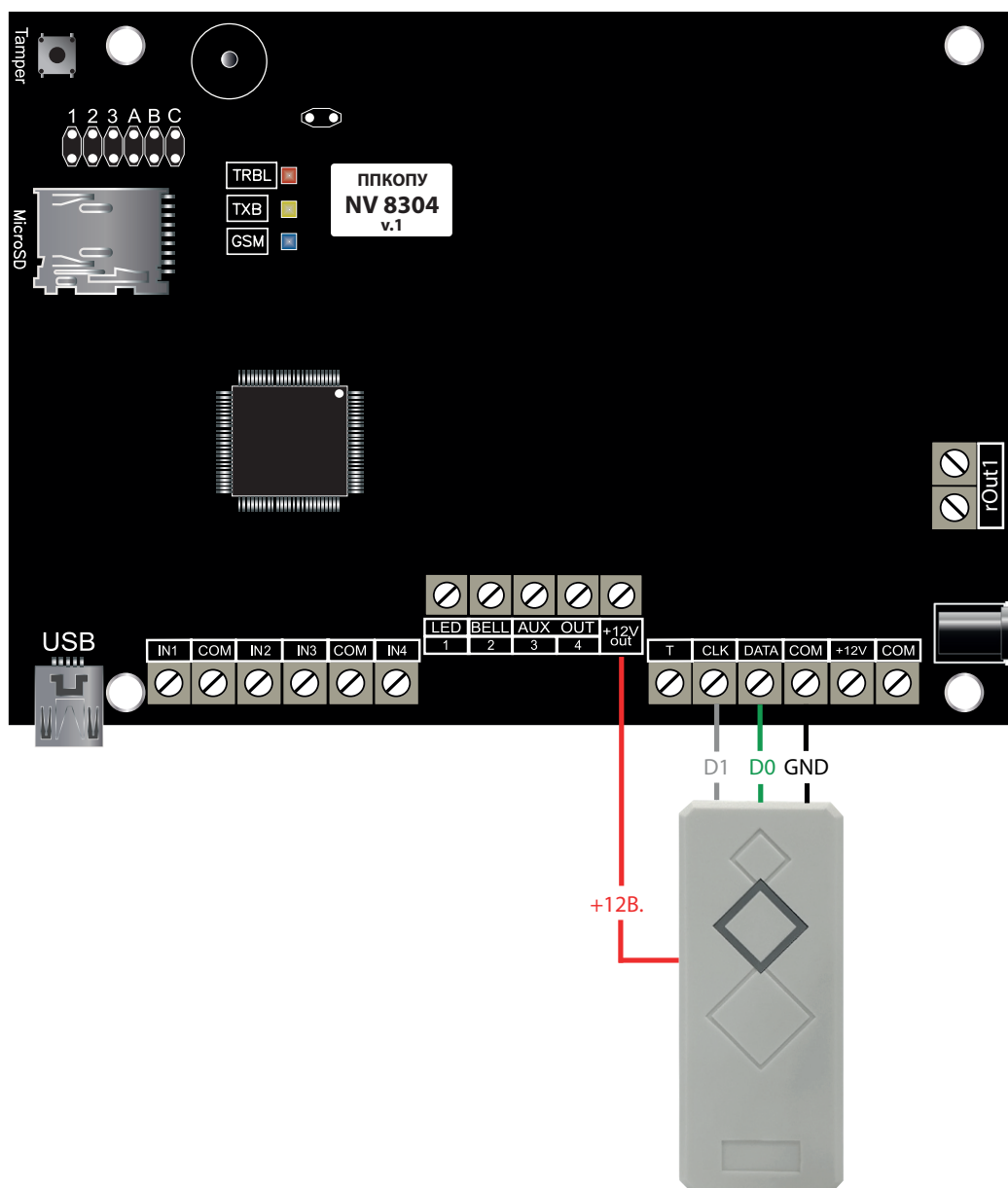
Схема подключения WG считывателя
