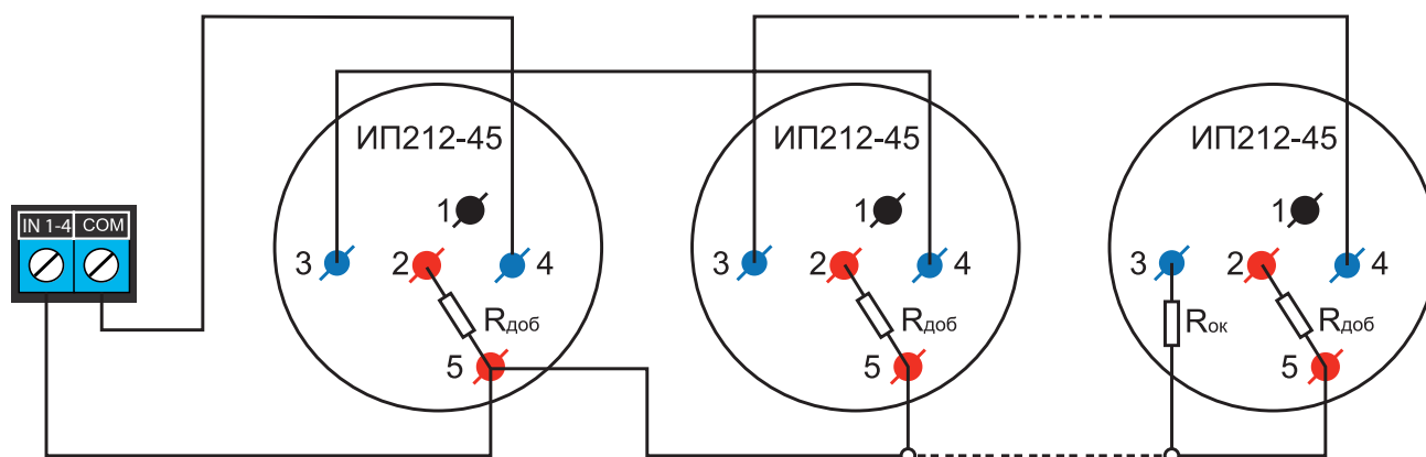
Схема подключения ИП212-45 к пожарному входу NV 8304 с добавочными и с оконечным резисторами
