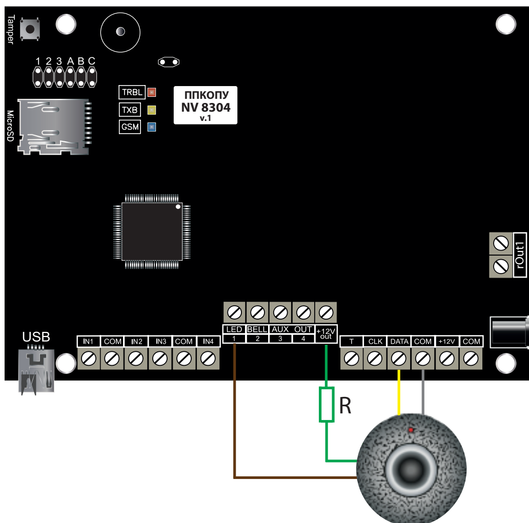
Схема подключения на примере ТМ считывателя STM-KT
