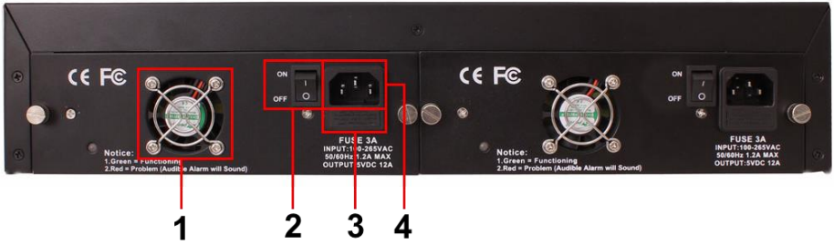
Рис. 3 Бокс О-142В, задняя панель
