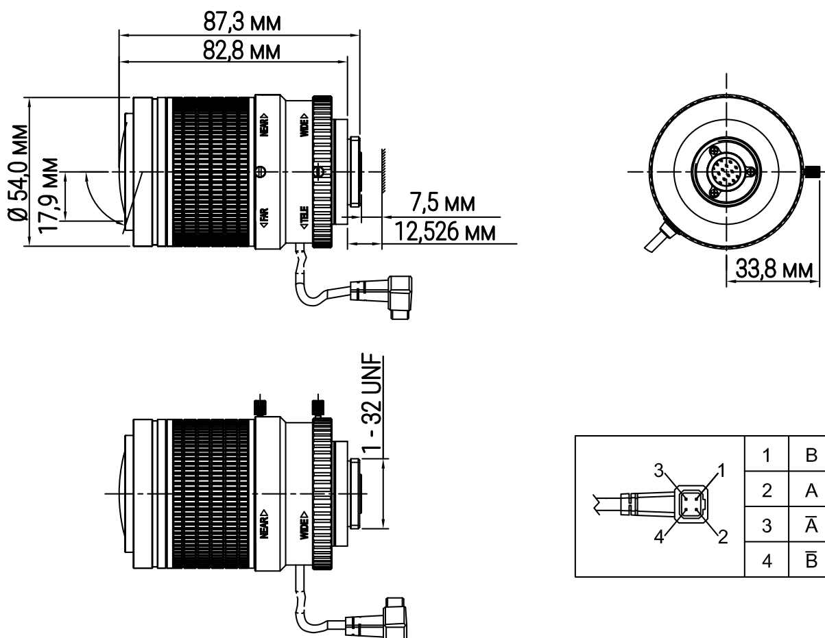
Рисунок 6.1 – Габаритные размеры
