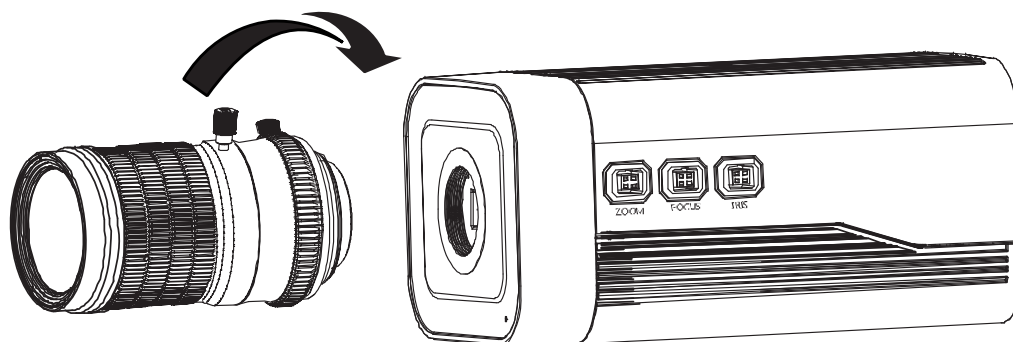
Рисунок 7.2 – Установка объектива
