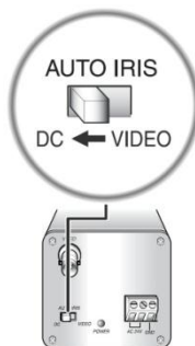
Рис.1. Переключатель Video/DC
