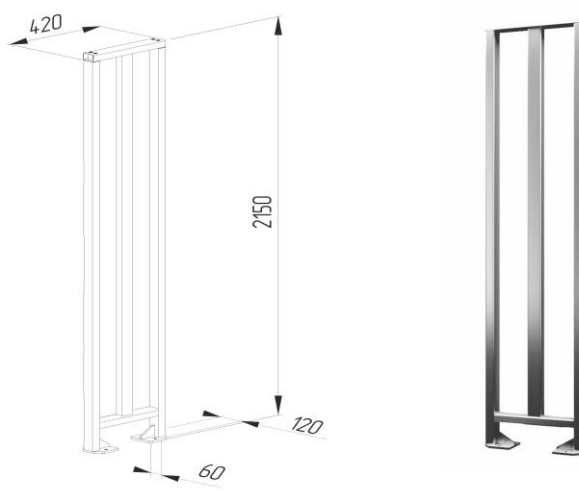
Ограждение полноростовое шириной 420мм
