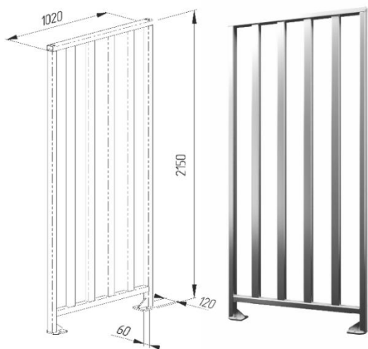
Ограждение полноростовое шириной 1020мм
