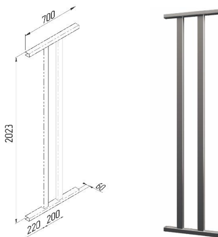
Дополнительная секция полноростового ограждения шириной 700мм
