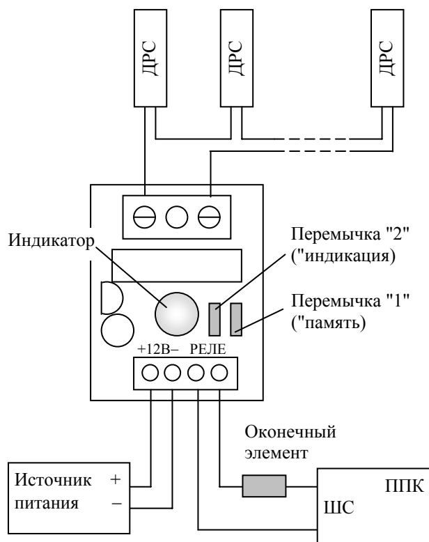
Схема подключения
