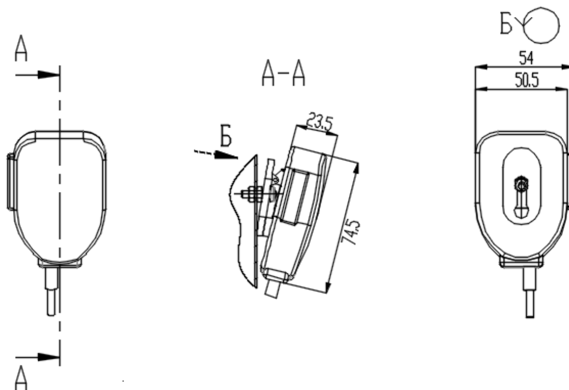
Рисунок 1 - Габаритный чертеж внешнего микрофона ВМ-03
