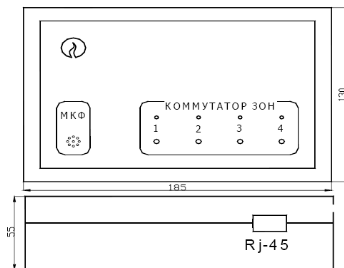
Рис.1. Общий вид ВПУ-4.
