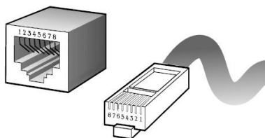
Рис. 10 Разъём RJ45 с пронумерованными контактами.
