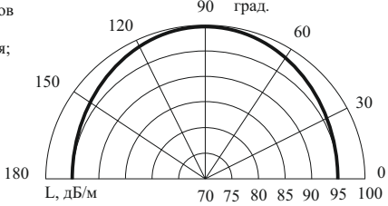
Рисунок 1 – Диаграмма направленности
