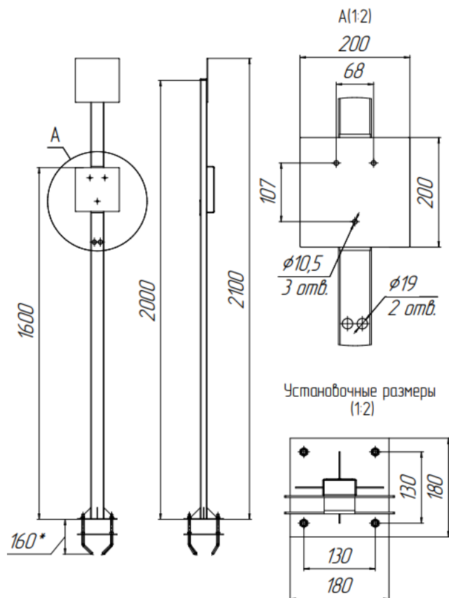
Рис.1 Стойка СП-03 «под бетонирование»
