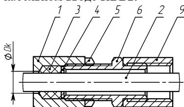
в) монтаж в трубной разводке с помощью штуцера ПШ
