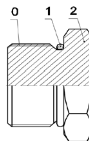
ЗАГЛУШКА – для глушения свободных отверстий под KB
