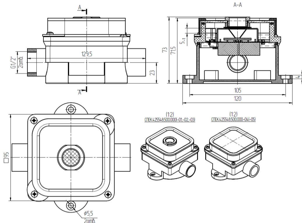
Рисунок А1 – Габаритные размеры оповещателя из полиамида
