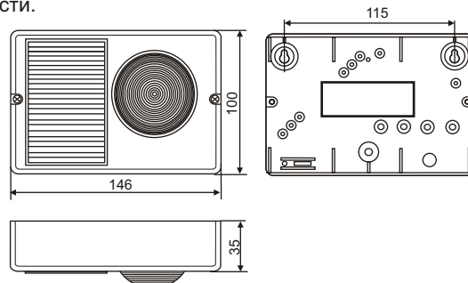
Рис.1. Габаритные и установочные размеры.
