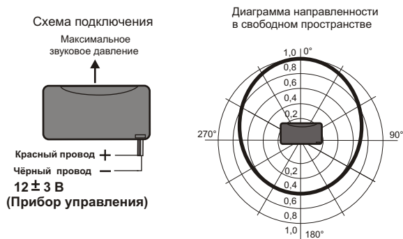
Рис.2 Схема подключения и диаграмма направленности звука оповещателя.
