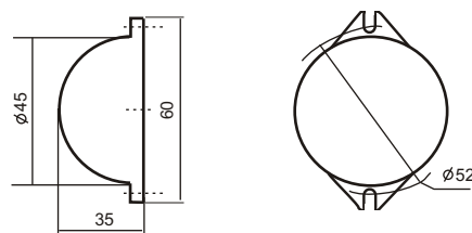
Рис.1. Габаритные и установочные размеры оповещателя
