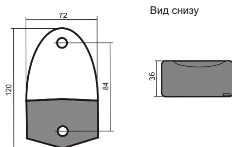
Рис.1. Габаритные и установочные размеры оповещателя
