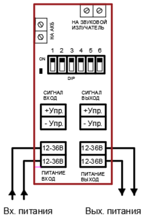
Рисунок Б1 – Схема 2-х проводного подключения оповещателя пожарного взрывозащищенного ТСВ 12÷36В. Номинал управляющего сигнала: 12÷36В DC, 12÷28В AC.
