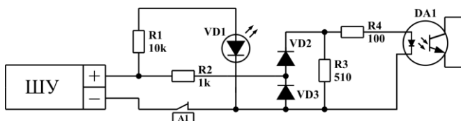
Рисунок 10. Схема каскада входа управления ШУ УЮО.
