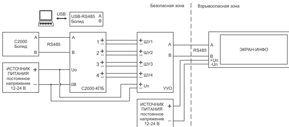
Рисунок 14. Пример подключения оповещателя ЭКРАН-ИНФО-RGB к блоку контрольно-пусковому C2000-КПБ через устройство управления УУО-RGB.
