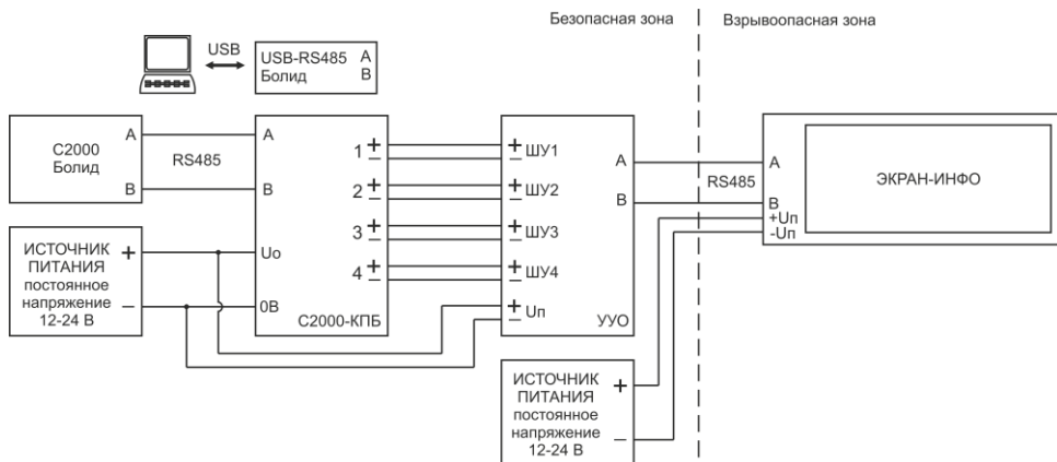
Рисунок 14. Пример подключения оповещателя ЭКРАН-ИНФО-RGB к блоку контрольно-пусковому С2000-КПБ через устройство управления УУО-RGB.
