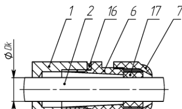
е) монтаж в кабельном вводе KBП12
