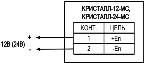
Рис.1. Схема подключения.
