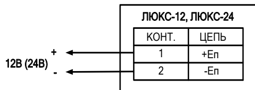
Рис.1. Схема подключения.
