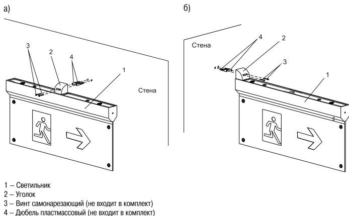
Рисунок 3 – Монтаж накладной
