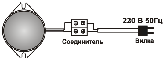
Рис.2 Схема подключения устройства “СБ-3”.
