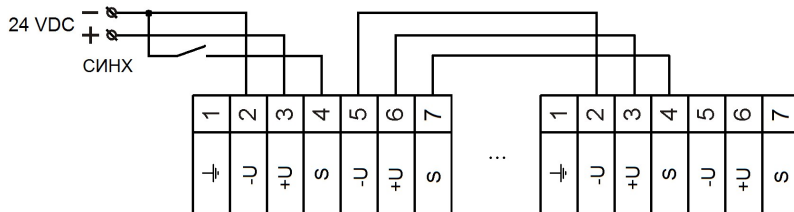
Рисунок 5. Внутренняя схема контроля цепи оповещателей BC-07e-Ex-3(I)-24VDC.
