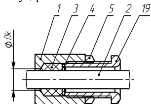
д) открытая прокладка кабеля в кабельном вводе KBВ
