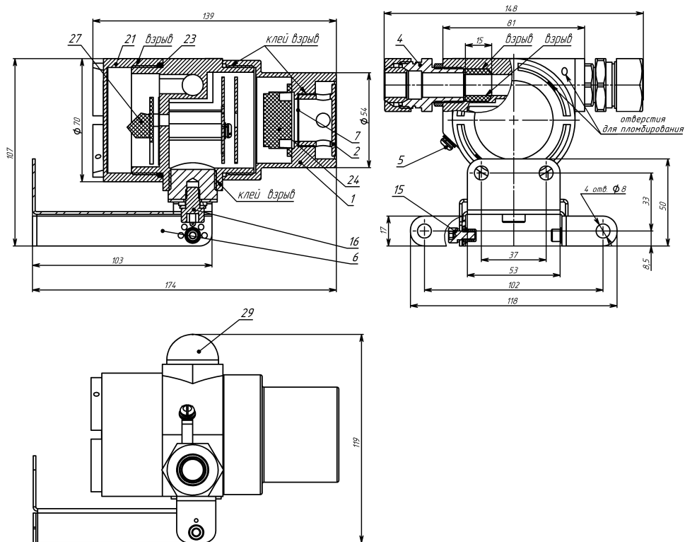
а) Габаритные размеры оповещателя ВС-07е-Ex-3(И).
