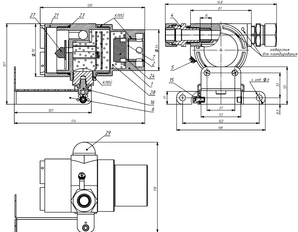
а) Габаритные размеры оповещателя ВС-07е-О-3(И).
