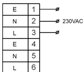
Рисунок 3. Схемы подключения оповещателей BC-07е-O-24VDC.
