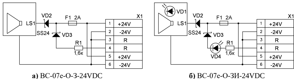
Рисунок 5. Внутренняя схема контроля цепи оповещателей BC-07е-O-3(И)-24VDC.
