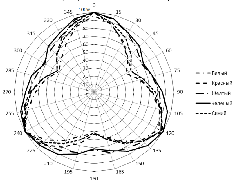
Рисунок 10. Нормированная диаграмма силы света ВС-07е-О-СД в зависимости от цвета колбы оповещателя.
