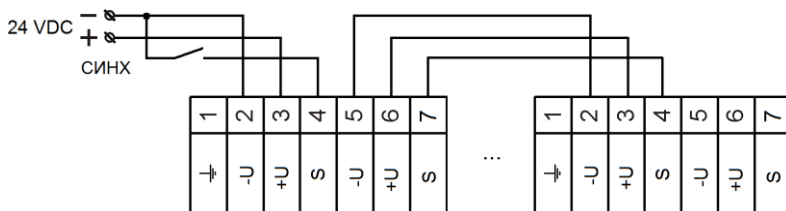
Рисунок 5. Внутренняя схема контроля цепи оповещателей BC-07e-O-3(И)-24VDC.
