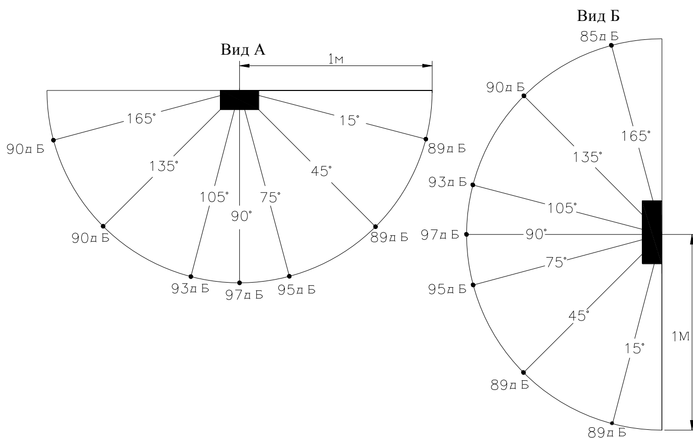
Рисунок 2.2.3.2 Диаграмма направленности звукового давления ОПЗ
