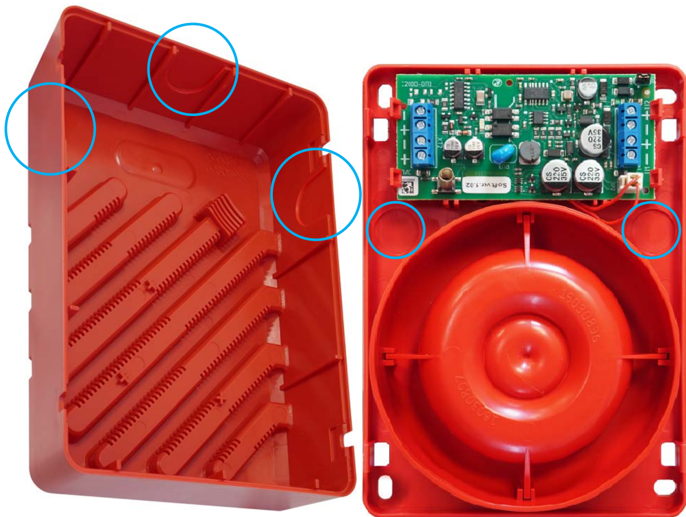
Рисунок 2.2.3.3 Места под выломы для ввода проводов ОПЗ
