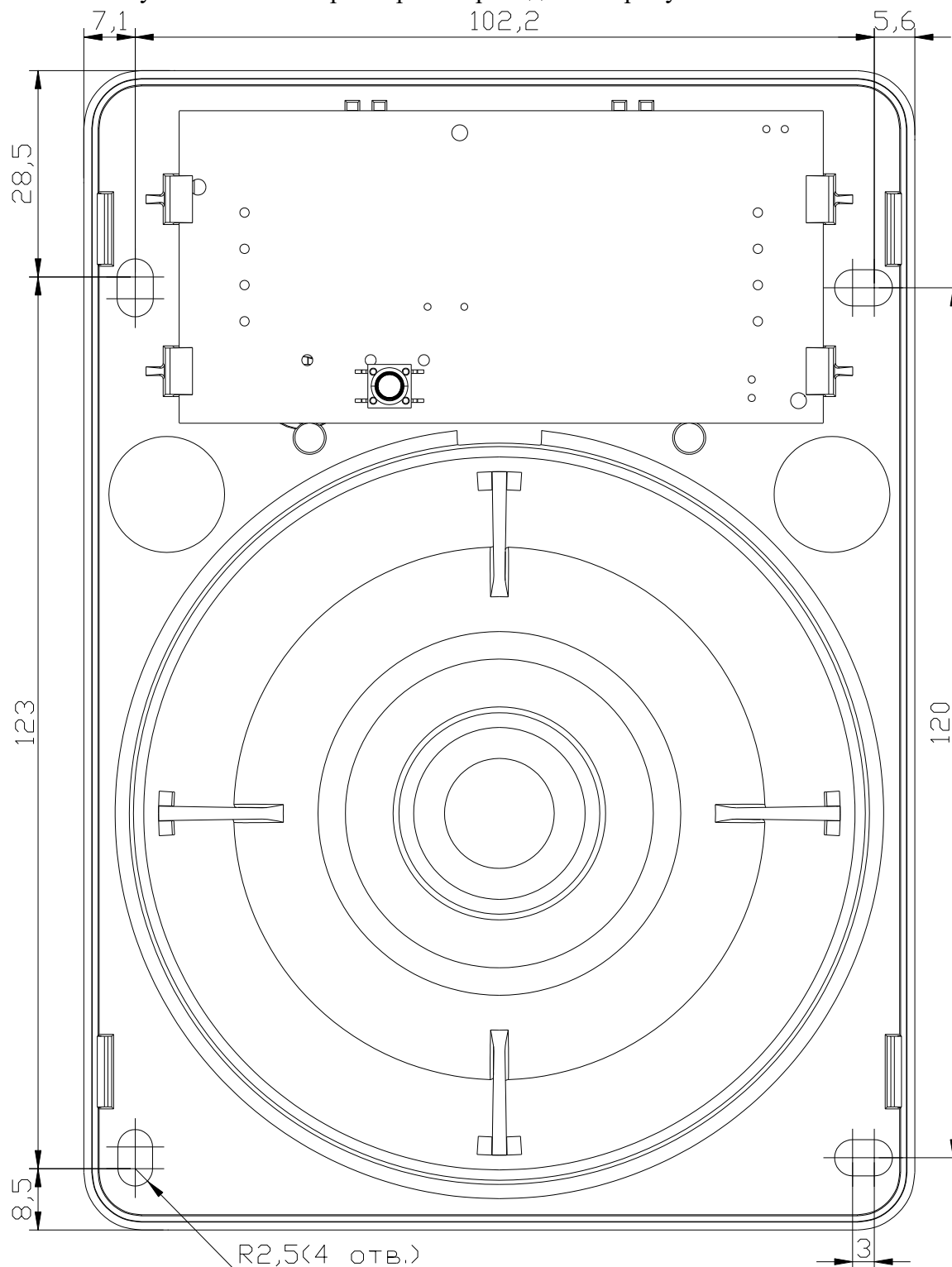
Рисунок 2.2.3.1 Установочные размеры ОПЗ
