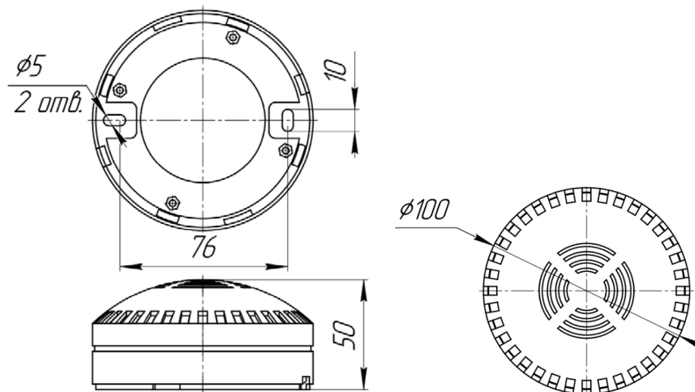
Рис.1 Габаритные и присоединительные размеры.
