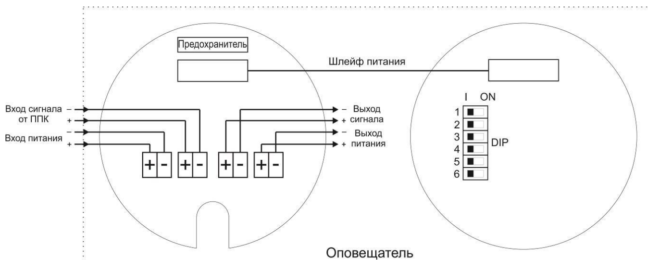
Рисунок 5 – Схема подключения оповещателя с питанием 12÷36 DC, 12÷28 AC. Номинал управляющего сигнала: 12÷36B DC, 12÷28B AC.
