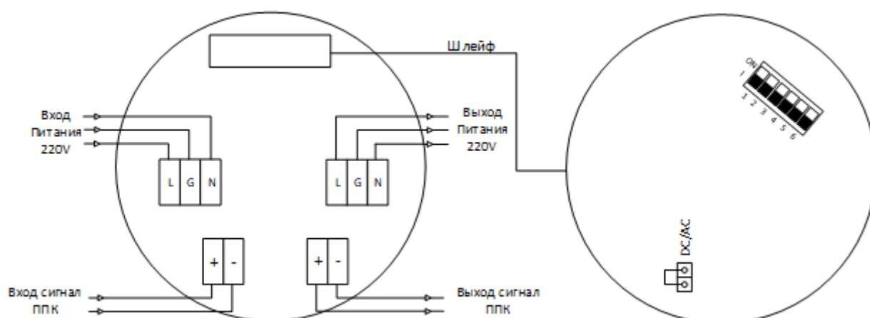
Рисунок Б2 – Схема подключения оповещателя с питанием 220В. Номинал управляющего сигнала: 12÷36В DC, 12÷28В AC.
