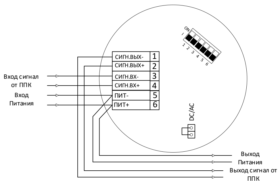
Рисунок Б1 – Схема подключения оповещателя с питанием 12÷36 DC, 12÷28 AC. Номинал управляющего сигнала: 12÷36В DC, 12÷28В AC.
