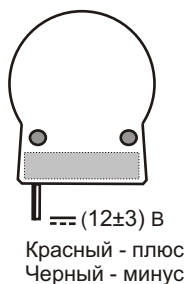
Рис.2 Схема подключения и диаграмма направленности оповещателя.
