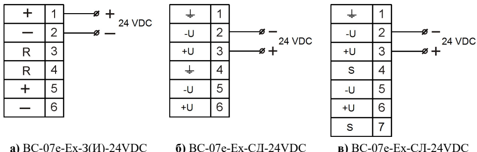
Рисунок 3. Схемы подключения оповещателей BC-07e-Ex-24VDC.
