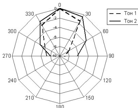
Рисунок 8. Диаграмма направленности звука BC-07e-Ex-3(I).
