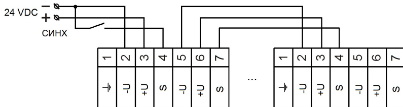
Рисунок 5. Внутренняя схема контроля цепи оповещателей BC-07e-Ex-3(И)-24VDC.
