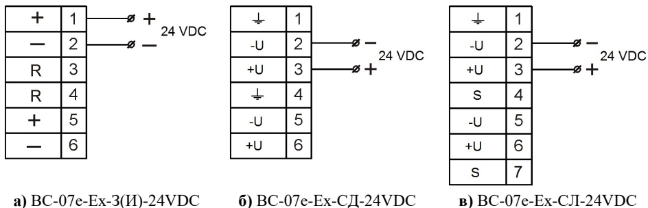
Рисунок 3. Схемы подключения оповещателей BC-07e-Ex-24VDC.
