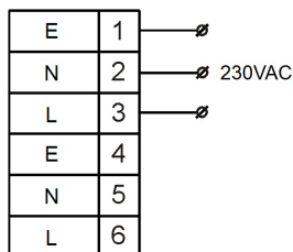
Рисунок 4. Схема подключения оповещателей BC-07e-Ex-230VAC.
