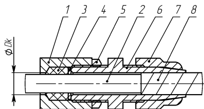
б) монтаж бронированным кабелем в кабельном вводе KBБ12
